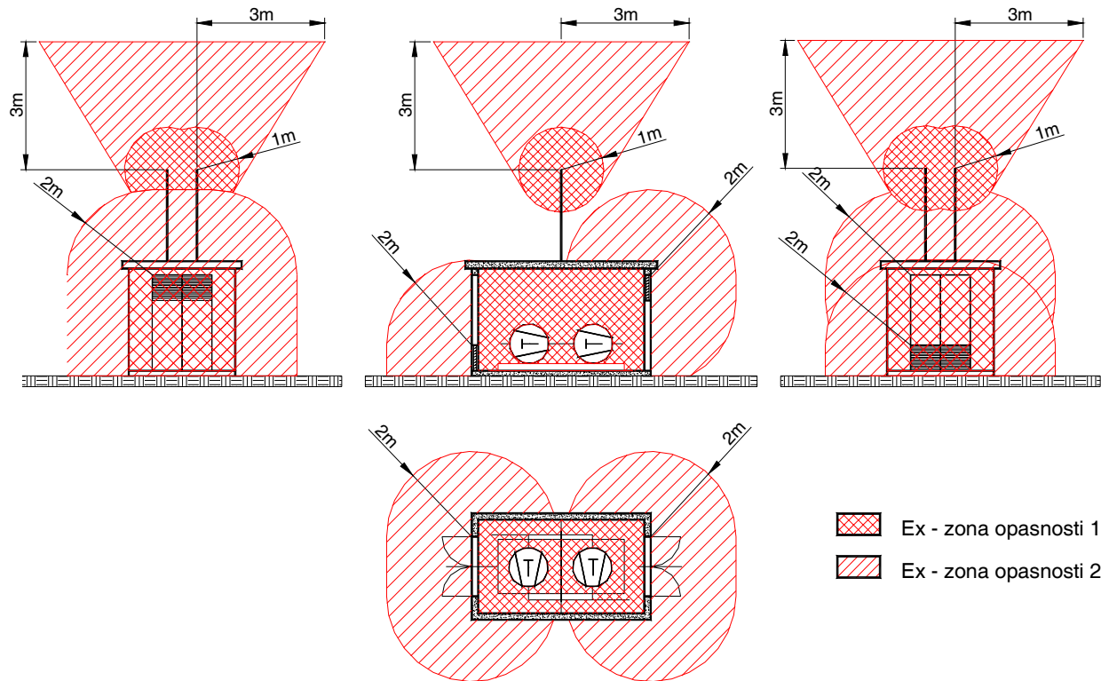
Sl. 2. Kompresorska jedinica smještena unutar građevine (zatvorenom području) - na internim postajama za opskrbu gorivom - bez sustava upozorenja prisutnosti plina
