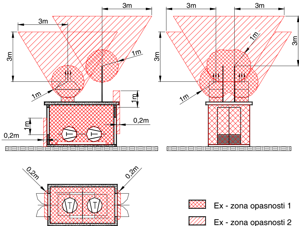
Sl. 3. Kompresorska jedinica smještena unutar građevine (zatvorenom području) - na javnim ili internim postajama za opskrbu gorivom - sa sustavom upozorenja prisutnosti plina
