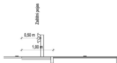
Slika 14. Zaštitni pojas biciklističke staze uz cestu izvan naselja sa zaštitnom ogradom
