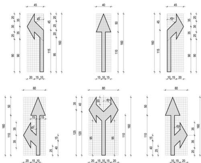
Slika 47. Izgled i dimenzije strelica na biclističkim površinama
