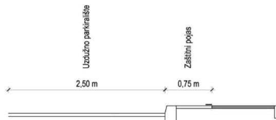
Slika 12. Zaštitni pojas biciklističke staze uz trak za uzdužno parkiranje
