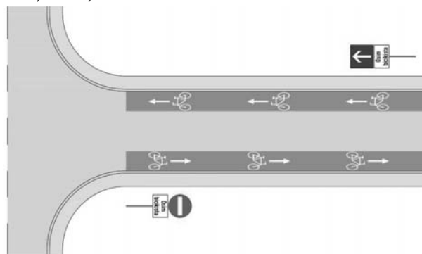
Slika 39. Izvedba obojanih biciklističkih traka u jednosmjernoj ulici
