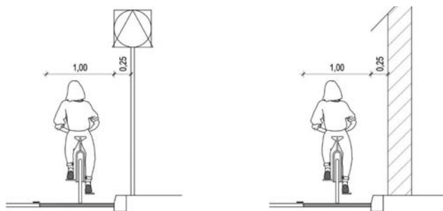
Slika 15. Širina zaštitnog pojasa biciklističke trake uz stalne zapreke
