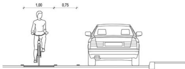
Slika 16. Širina zaštitnog pojasa biciklističke trake uz trak uzdužno parkiranje
