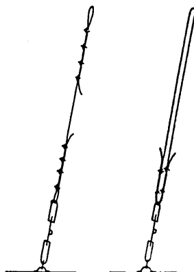
Slika 5: Alternativne izvedbe priveza od čeličnog užeta
